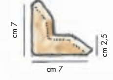
SQS / 7 spessore thickness cm 1,7
