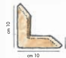
SQS / 10 spessore thickness cm 1,7
